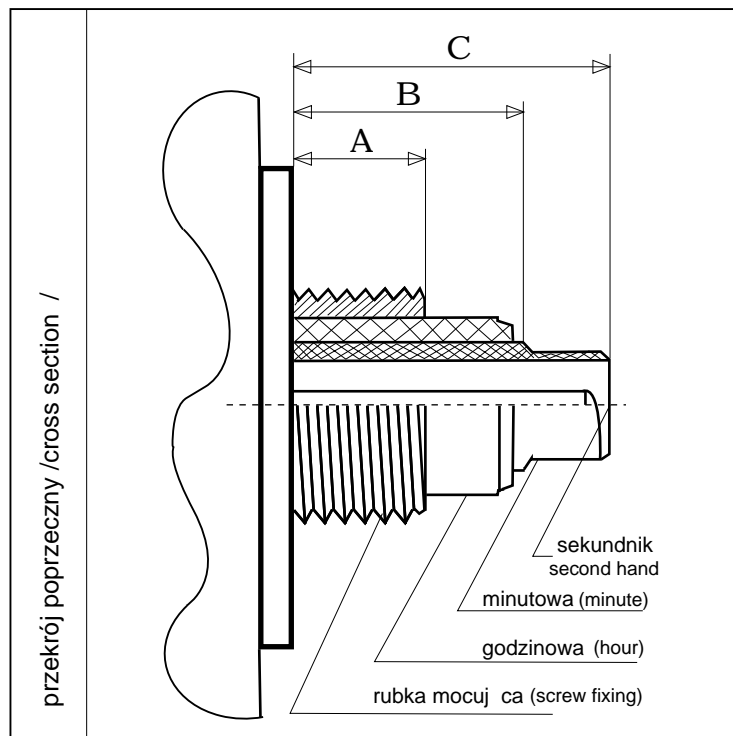
Diagram: Trzpie słu cy do mocowania zarówno mechanizmu jak i wskazówek Movement shaft for mounting movement and hands Вал передвижения фиксации стрелки и механизм
